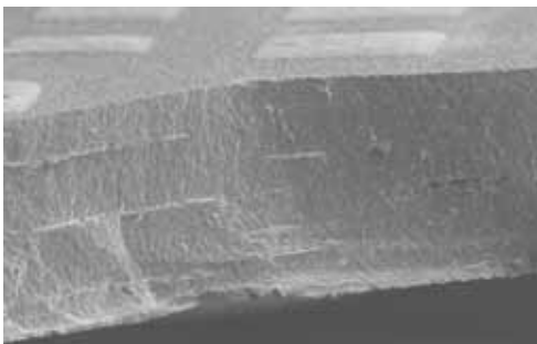
Bruchfläche durch eine keramische Leiterplatte im Raster-elektronenmikroskop. Die metallischen Leiterbahnen und Kontakte sind zu erkennen.
